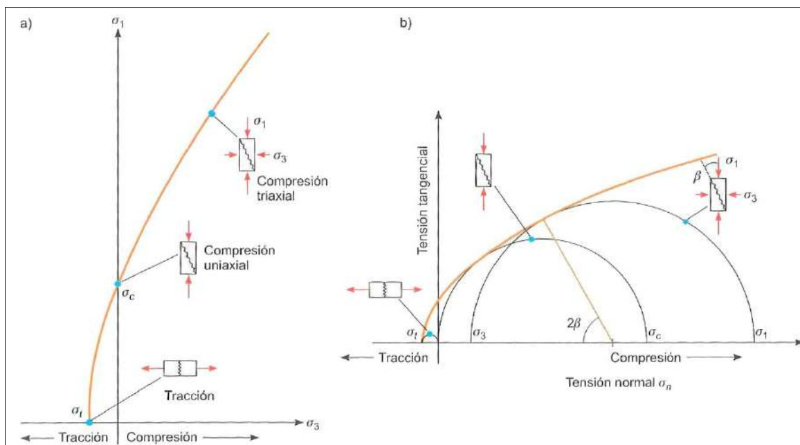
Figura 2. Envoltentes de rotura del criterio de Hoek-Brown en función de los esfuerzos principales (a) y de los esfuerzos normales y tangencial (b). Representación de las diferentes condiciones de (González et al., 2003)
