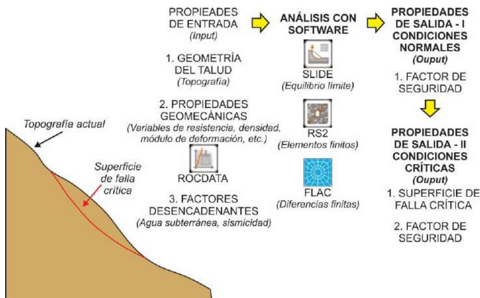
Figura 16. Metodología del análisis de inestabilidad de las laderas y taludes críticos en la investigación.
