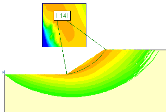
Figura 9. Círculo de falla crítica según su factor de seguridad en Slide. (Rocscience, 2016).
