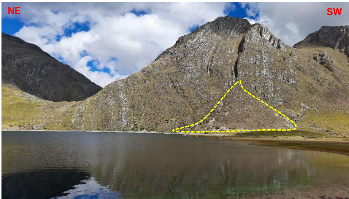
Foto 24. Geofoma denominada Cono de Derrubio en material carbonático en cerros circundante a la Laguna.
