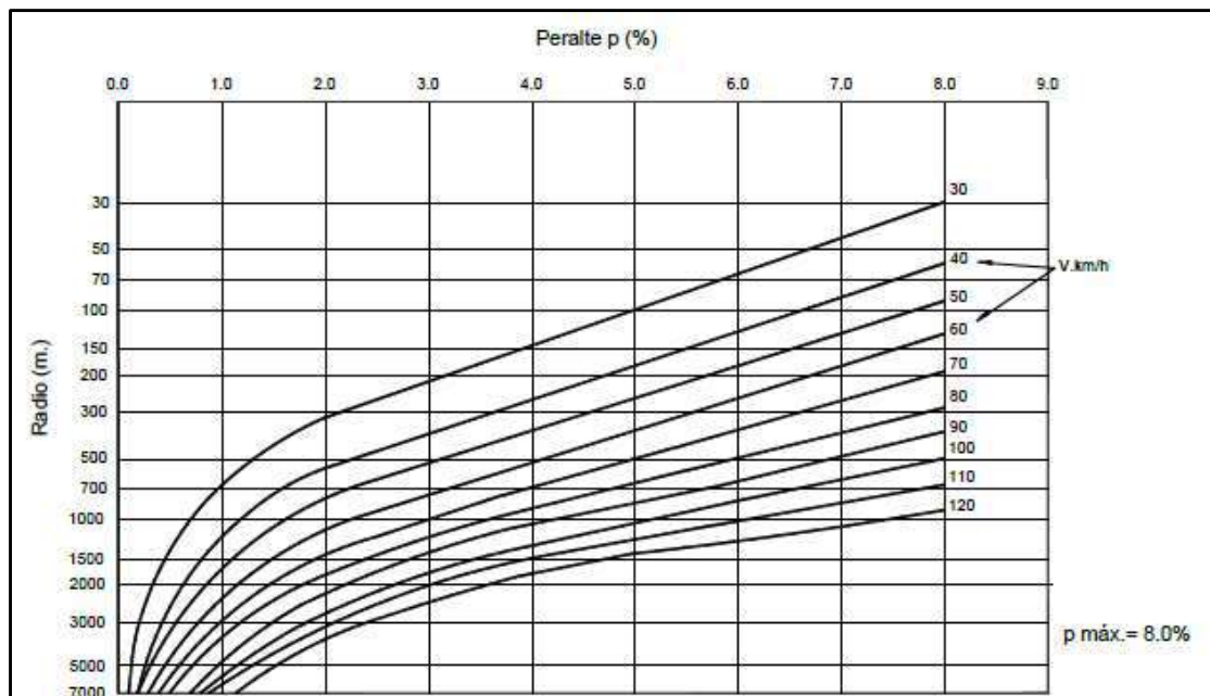
Figura 4.7. Peralte en zona rural (Tipo 1, 2 ó 3).
