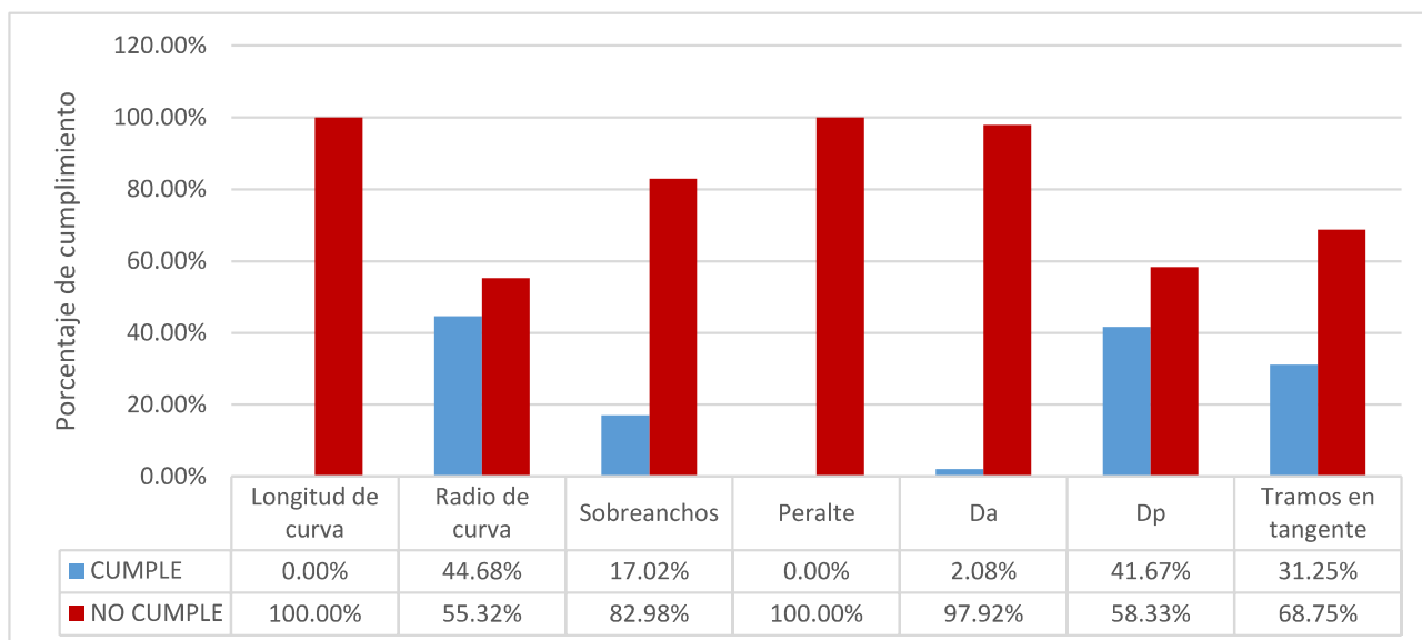
Figura 4.17. Verificación de parámetros en planta.
