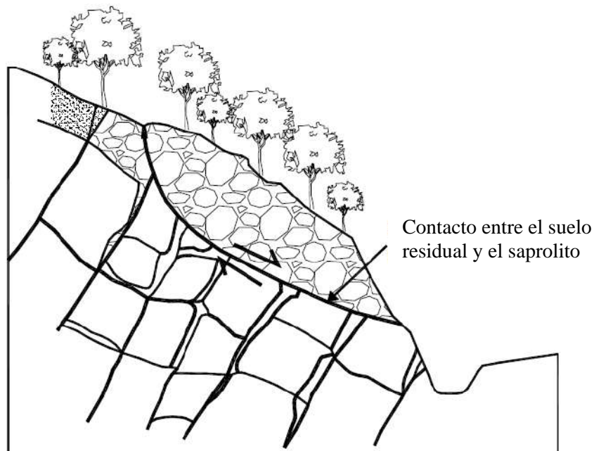
Figura 6. Deslizamiento compuesto, que inicia en el suelo residual (menos resistente), profundiza hasta el saprolito (más resistente) y sigue la discontinuidad.
