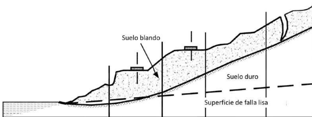
Figura 5. Deslizamiento de traslación. Fuente: Tomado de Suárez, (2009).
