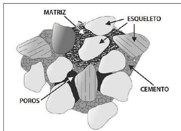
Figura 2. Esquema de estructuración de una roca detrítica (Arribas, 2010)
