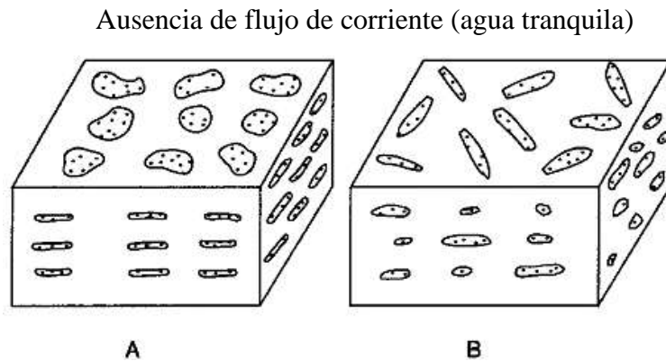
Figura 9. A. Granos laminares o escamosos depositados en agua tranquila sobre un lecho plano. B. Granos alargados depositados en disposición aleatoria en aguas tranquilas. Tomado de (Boggs, 2009).
