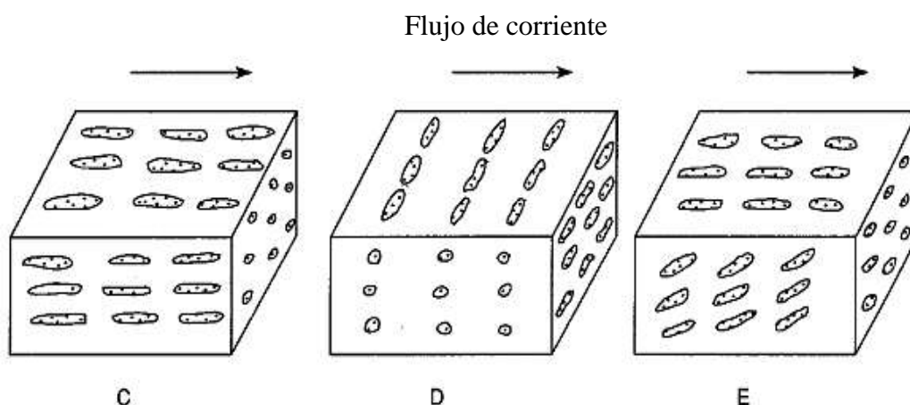
Figura 10. Disposición hipotética y esquemática de granos en sedimentos. C. Granos alargados depositados bajo el flujo de corriente con dimensiones largas paralelas al flujo de corriente. D. Granos alargados depositados bajo el flujo de corriente con dimensiones largas perpendiculares al flujo de corriente. E. Granos alargados depositados en un arreglo imbricado bajo el flujo de corriente. Tomado de (Boggs, 2009).
